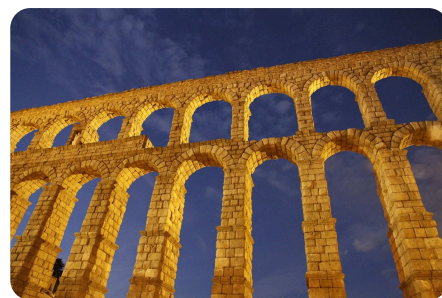
Acueducto de Segovia (fines del s. I o comienzos del II d. C.): granito sin argamasa, 28 m de altura máxima. Las obras públicas romanizaron el territorio. Foto: David Corral Gadea (CC BY-SA 3.0 ES).
