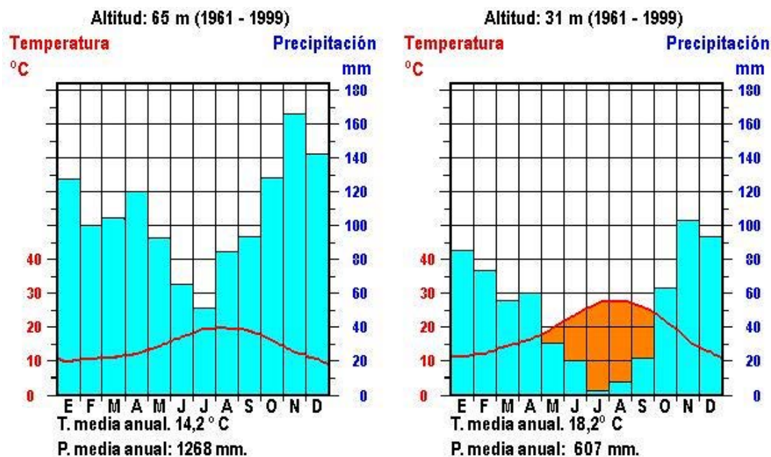
Climogramas de dos observatorios meteorológicos españoles como ejemplos de climas en España
